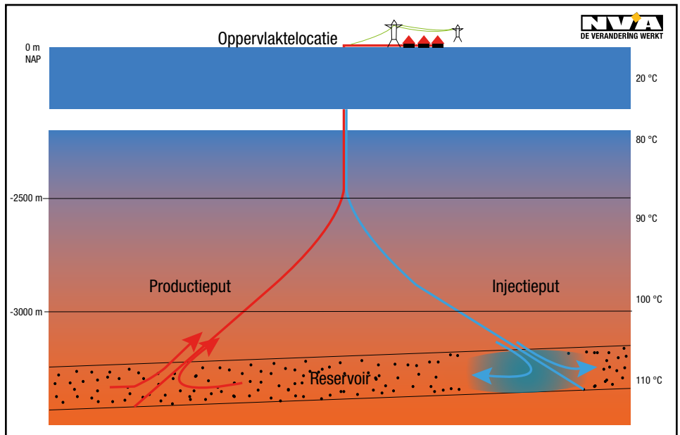
Afbeelding: Schematische voorstelling van de geothermische werking. (naar grafiek: EarthlyMatters)
